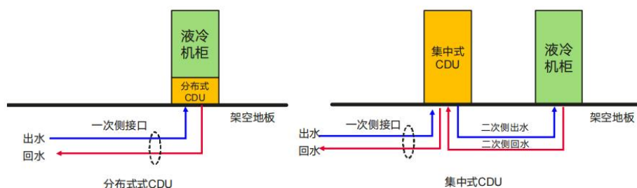
图9：集中式和分布式 CD 示意图
