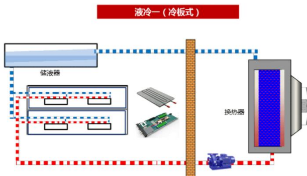
图 11：冷板式液冷工作原理
