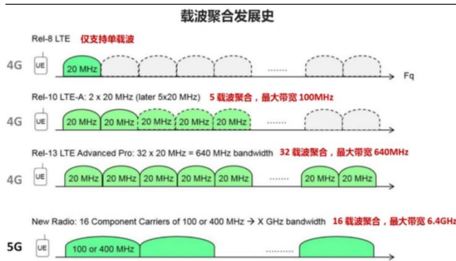
图3：载波聚合发展史
